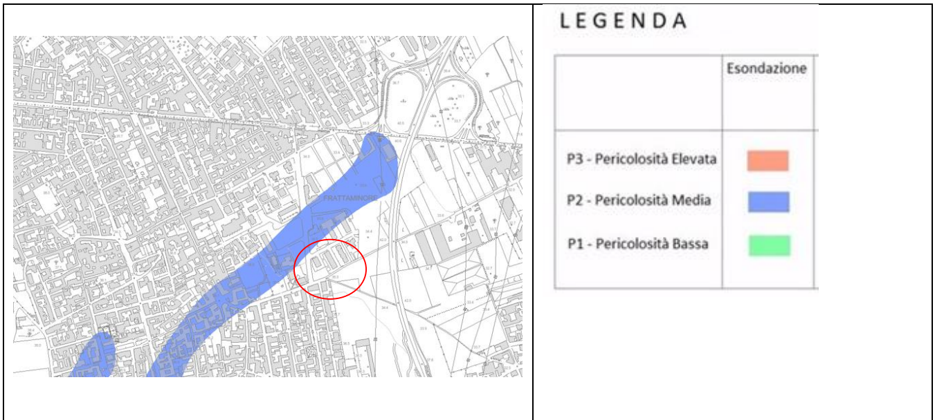
Stralcio della carta della pericolosità per fenomeni di allagamento da esondazione dell’Autorità di Bacino Nord Occidentale della Campania.
