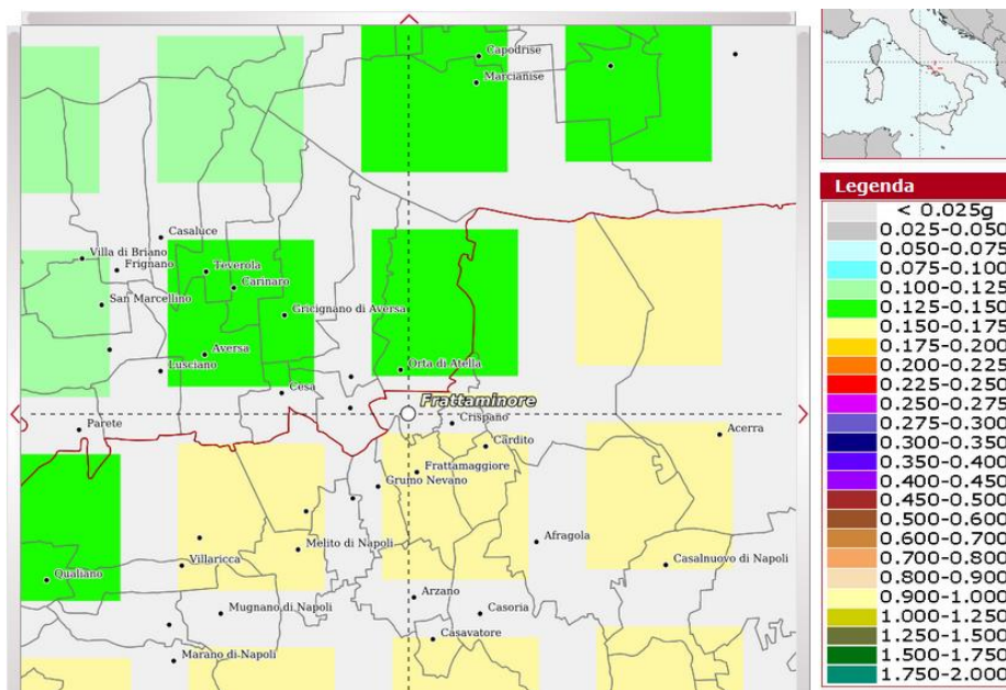
Mappa della pericolosità sismica del territorio comunale di Frattamaggiore (NA) dell'INGV con i range di valori delle ag nella legenda corrispondente
