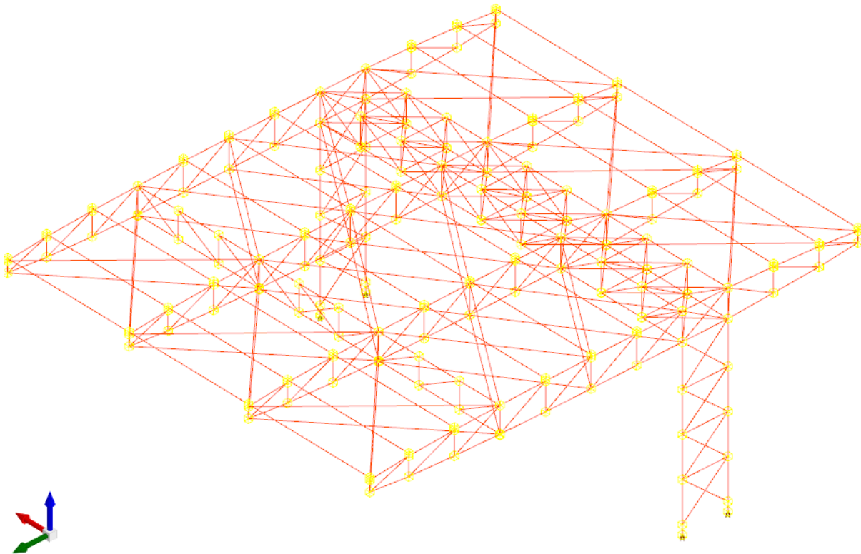
Figura 3. Modello analitico
