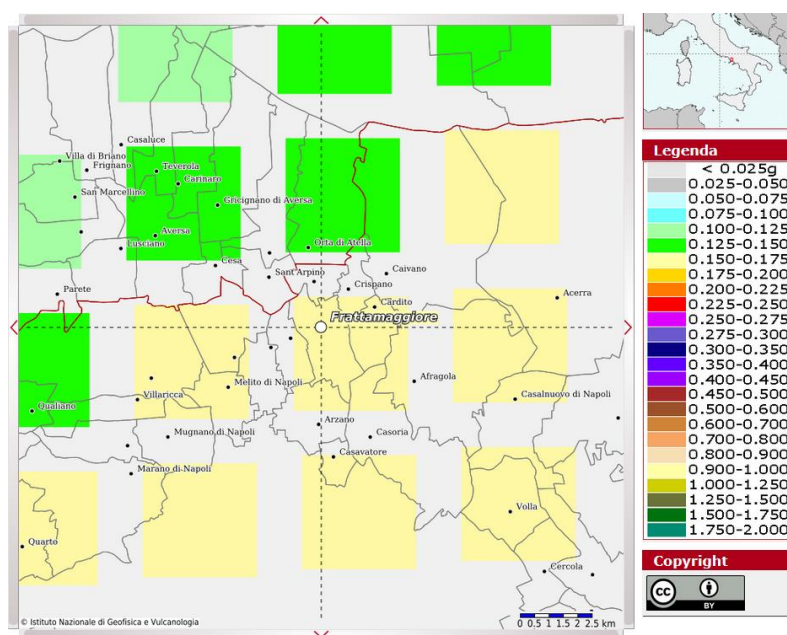
Mappa della pericolosità sismica del territorio comunale di Frattamaggiore (NA) dell'INGV con i range di valori delle ag nella legenda corrispondente
