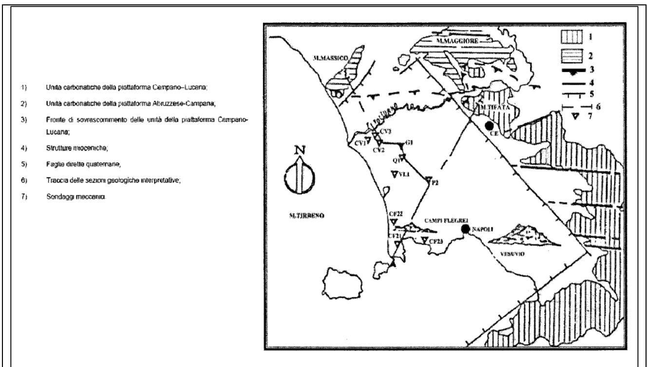
Fig. 3 –Schema tettonico della Piana campana
