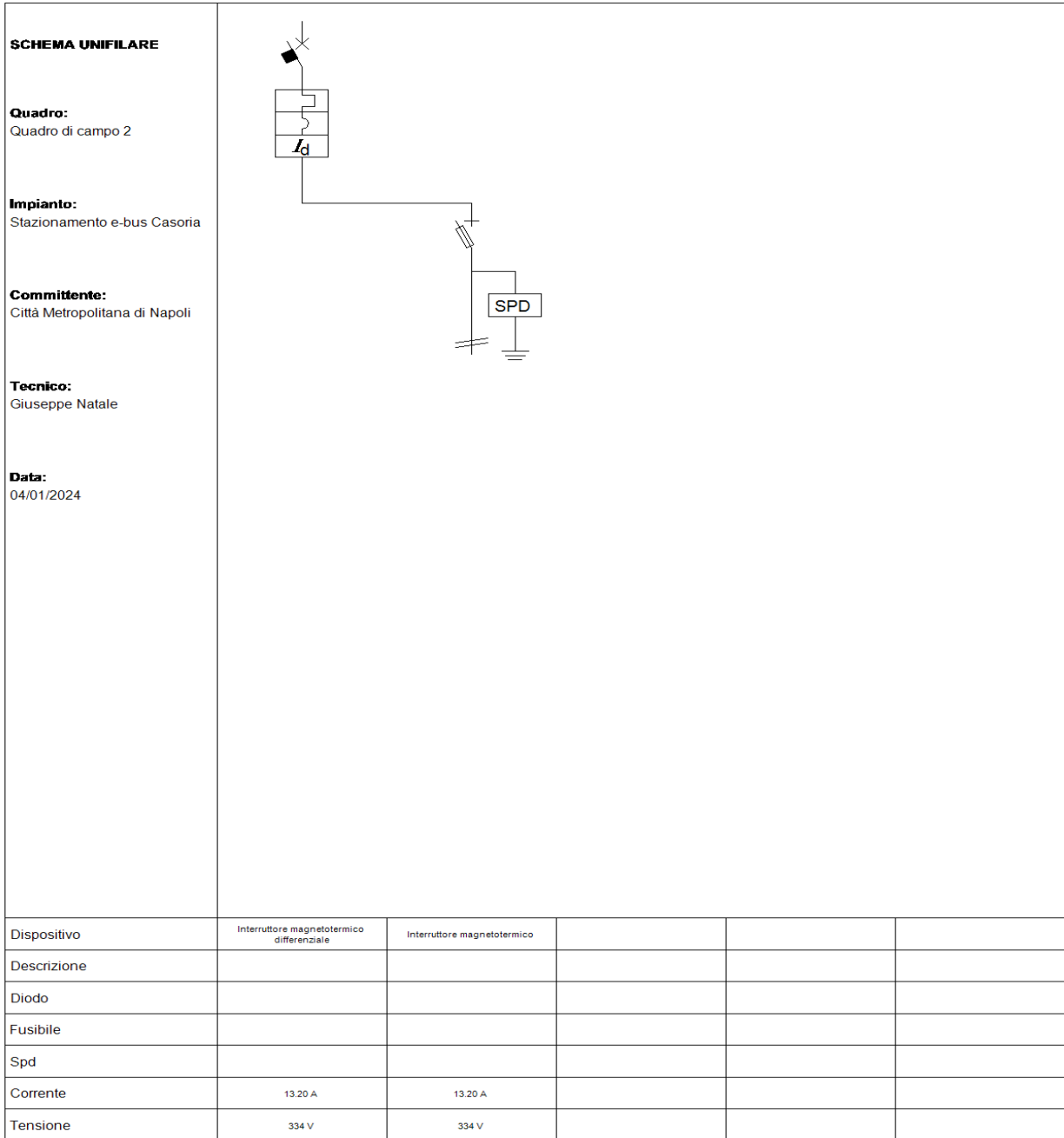
Fig. 7: Schema unifilare quadro "Quadro di campo 2"
