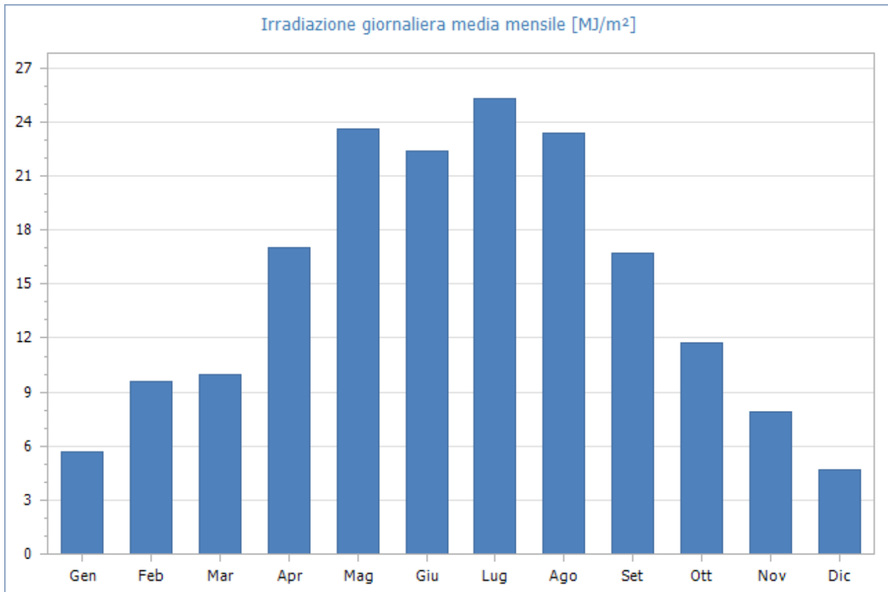
Fig. 1: Irradiazione giornaliera media mensile sul piano orizzontale [MJ/m 2 ]- Fonte dati: UNI 10349:2016 - Stazione di rilevazione: Airola
