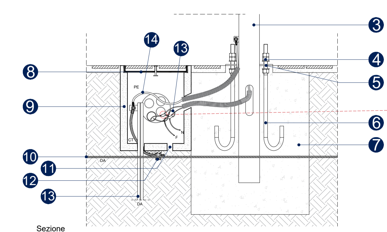
Dettaglio derivazione in pozzetto
