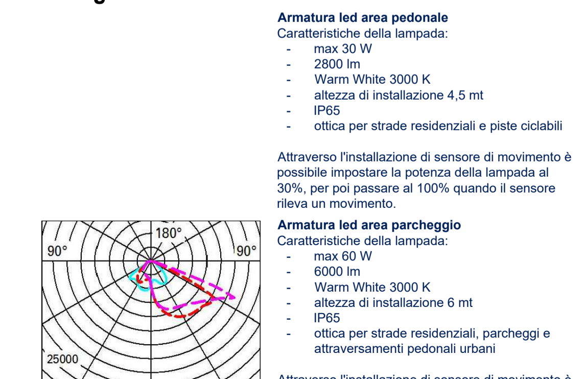
Dettaglio armatura led
