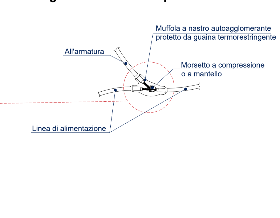
Dettaglio derivazione in pozzetto
