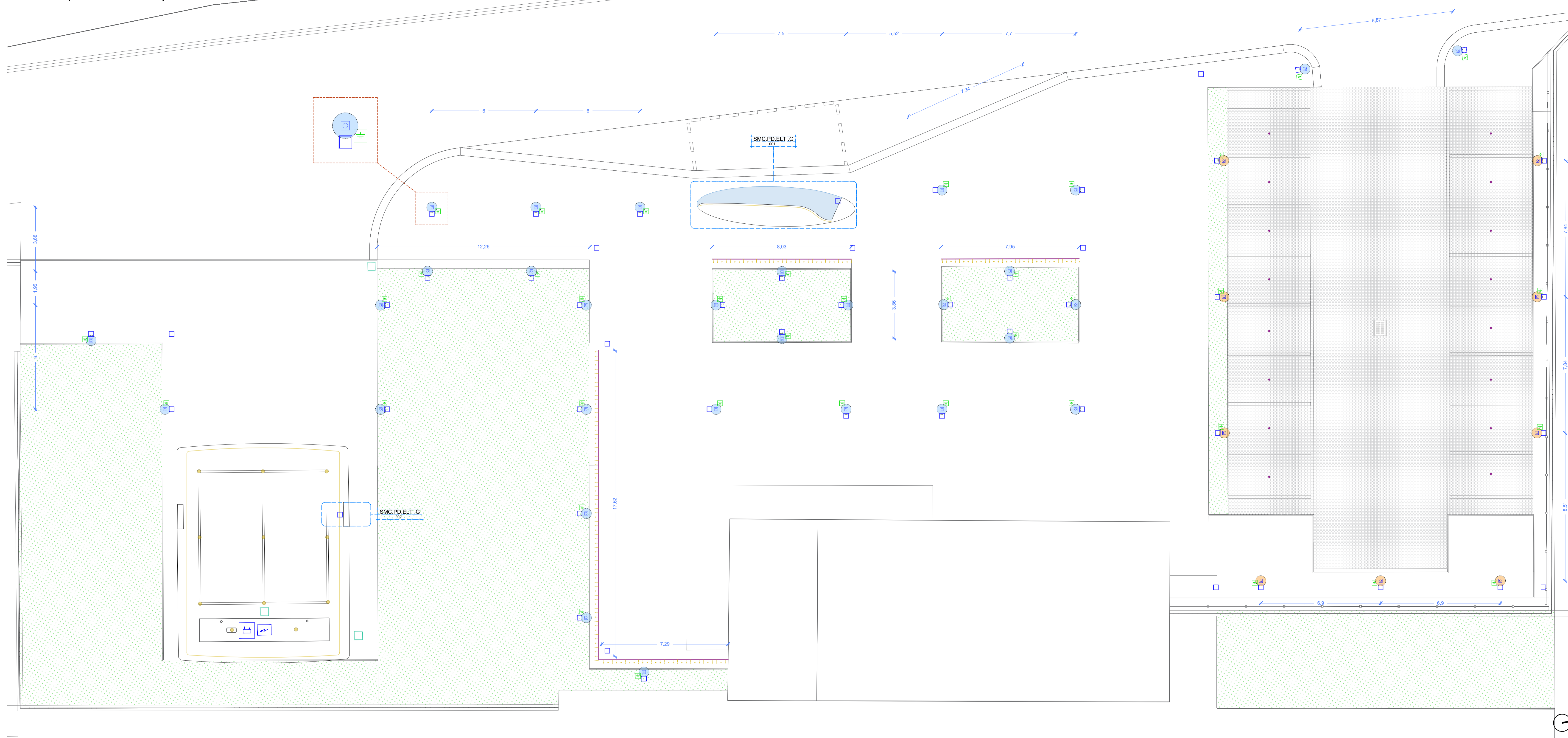
Planimetria posizionamento corpi illuminanti - scala 1:100
