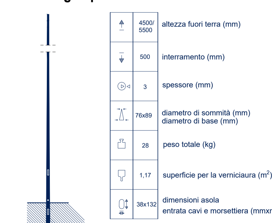
Dettaglio palo
