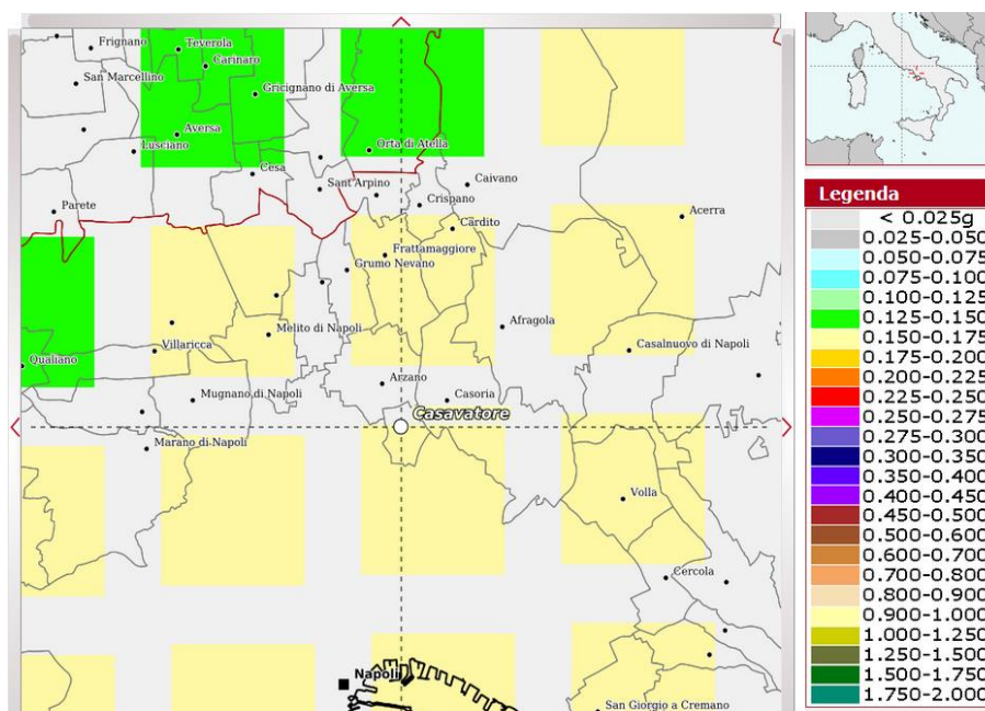
Mappa della pericolosità sismica del territorio comunale di Casavatore (NA) dell'INGV con i range di valori delle ag nella legenda corrispondente
