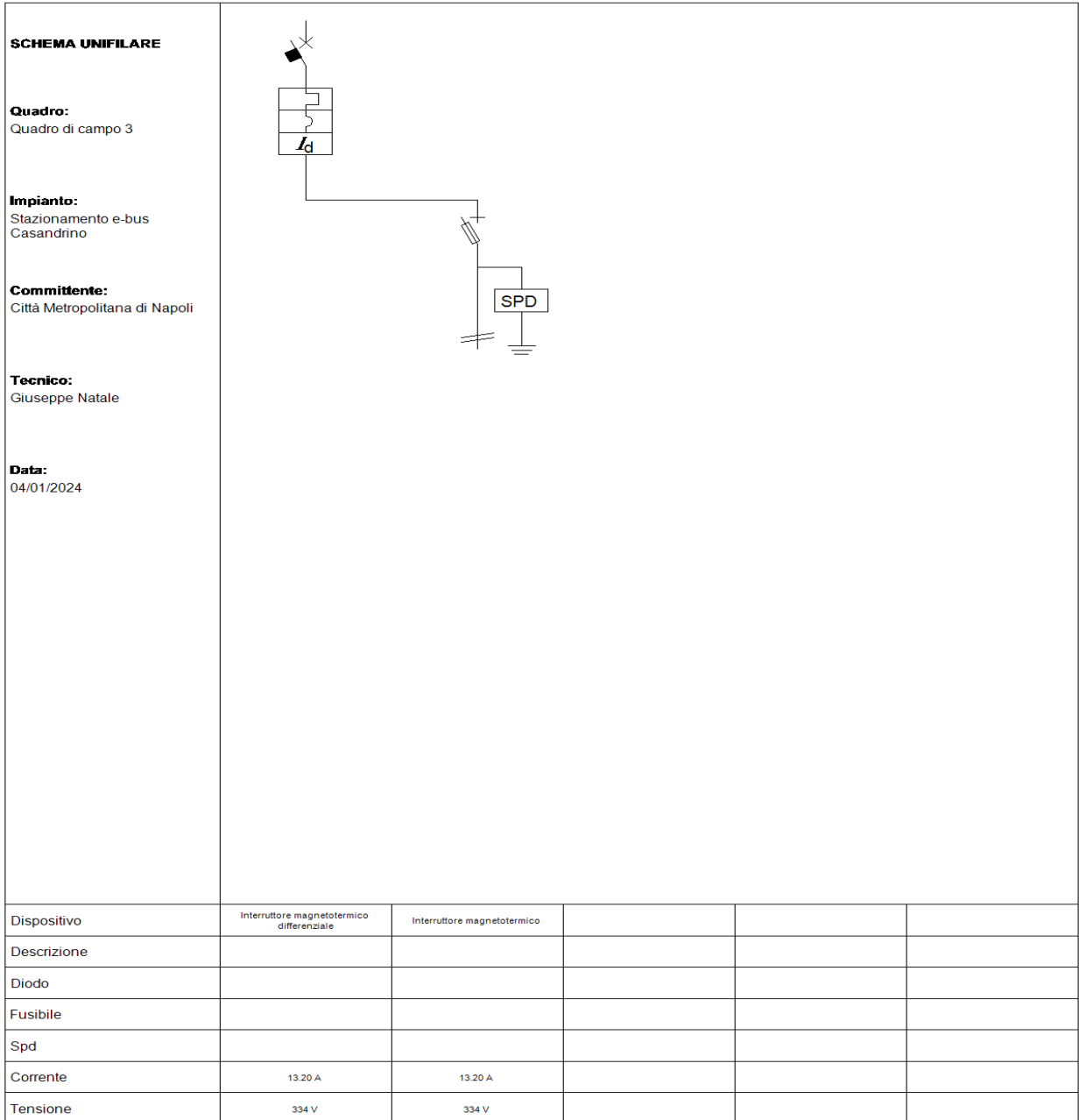
Fig. 8: Schema unifilare quadro "Quadro di campo 3"
