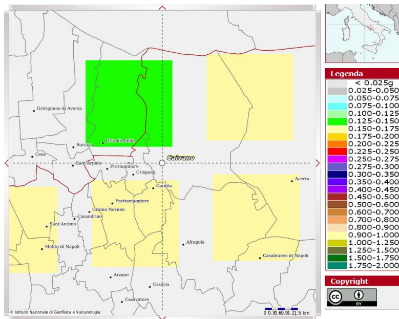
Mappa della pericolosità sismica del territorio comunale di Caivano (NA) dell'INGV con i range di valori delle a_g nella legenda corrispondente
