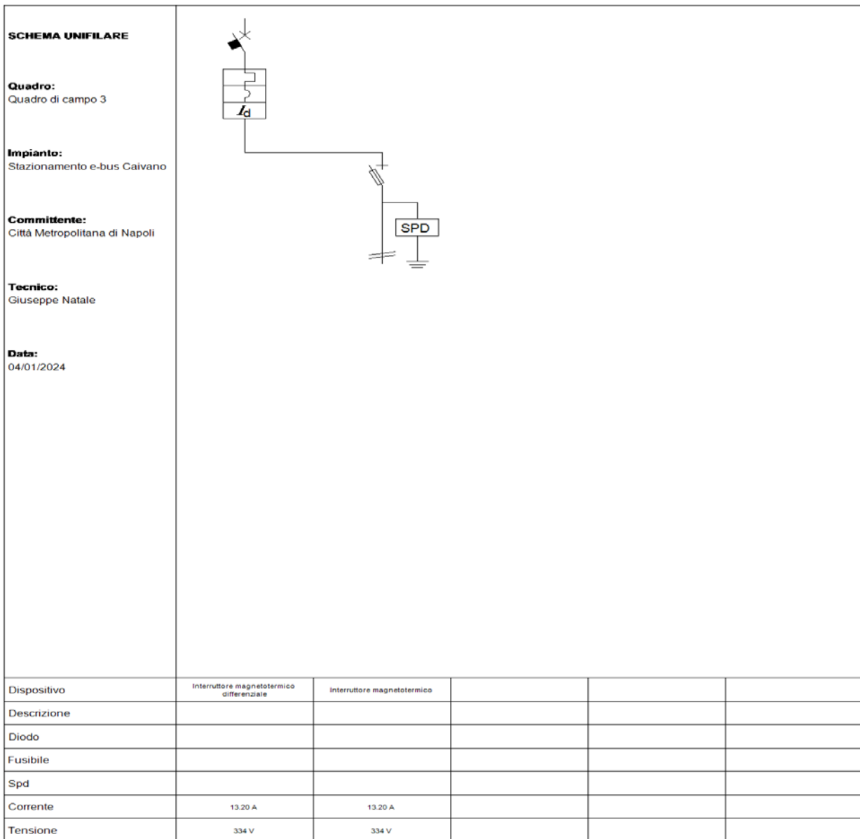
Fig. 8: Schema unifilare quadro "Quadro di campo 3"
