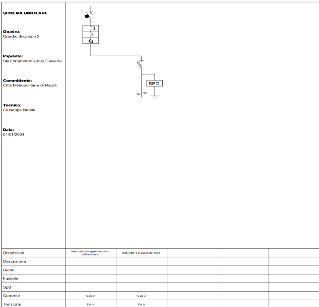
Fig. 7: Schema unifilare quadro "Quadro di campo 2"
